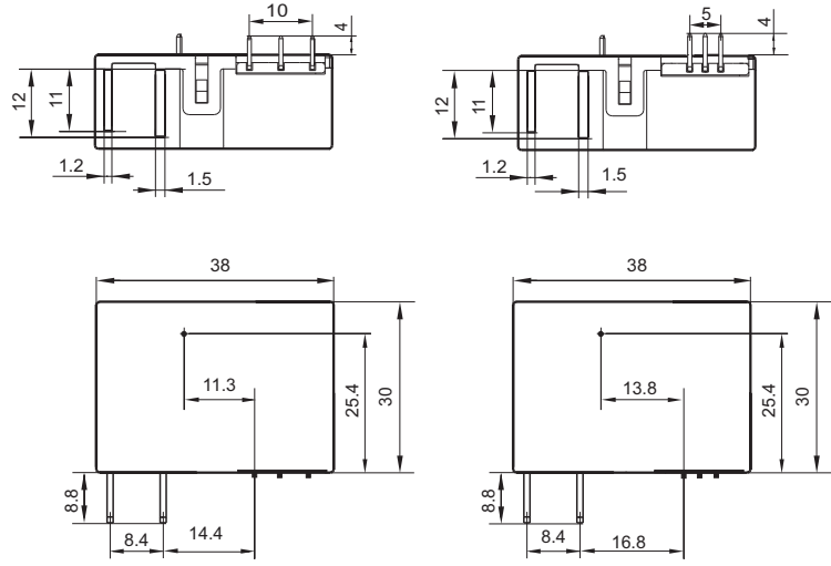
安装孔尺寸(底视图)
